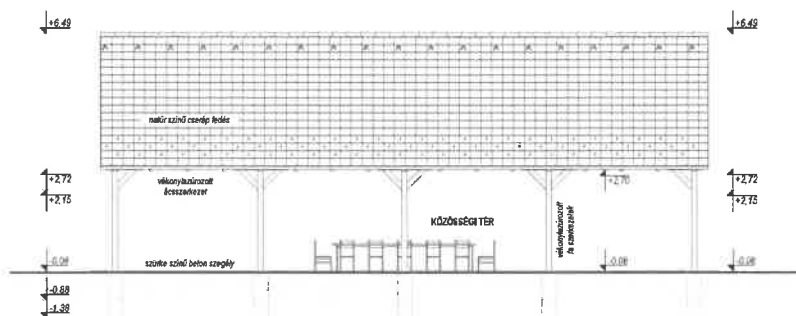
DÉL-NYUGATI HOMLOKZAT M 1.100
