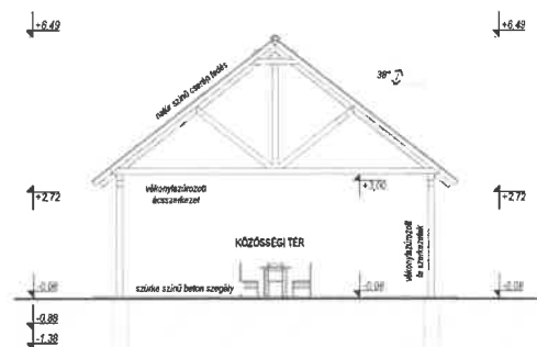
DÉL-KELETI HOMLOKZAT M 1.100
