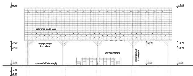
ÉSZAK-KELETI HOMLOKZAT M 1.100
